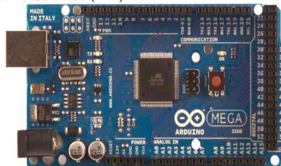
Fig1. Arduino MEGA
