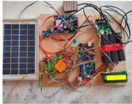
Fig12. LCD Displaying Latitude and Longitude
